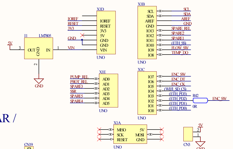
ARDUINO UNO
