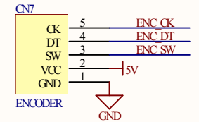
ENCODER
