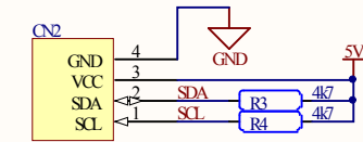
LCD (I2C)
